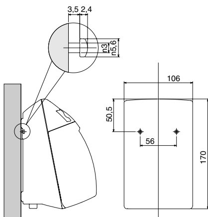
Haken für Wandmontage
