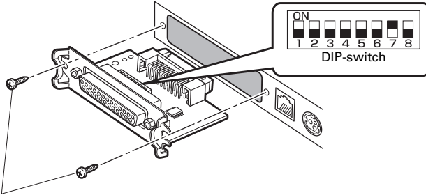
Viti di fissaggio della scheda d'interfaccia seriale
