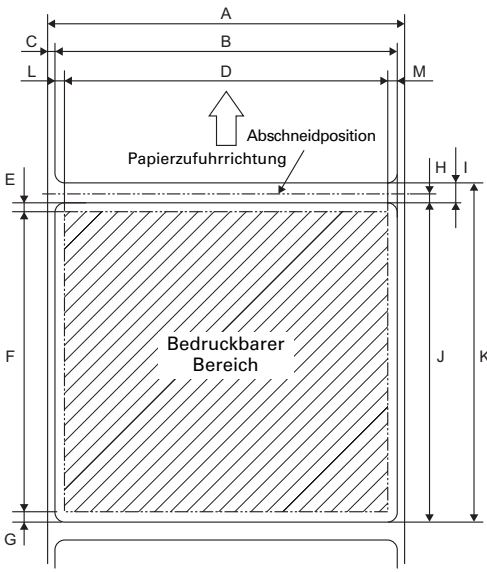
Papierrollen-Spezifikationen
