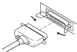
Interface parallèle
