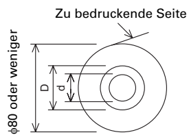
Papierrollen-Spezifikationen
